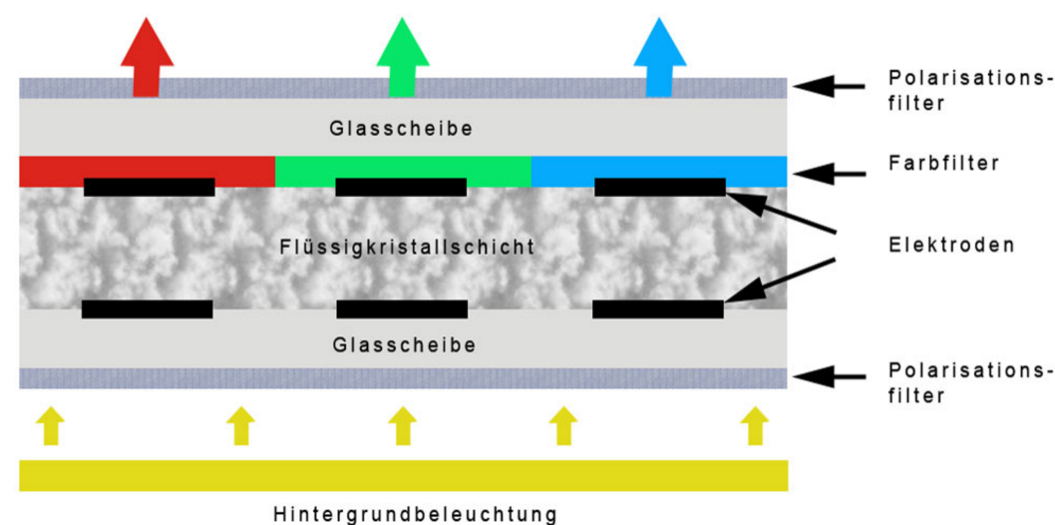
Fig 1. Schematischer Aufbau eines LC-Displays
